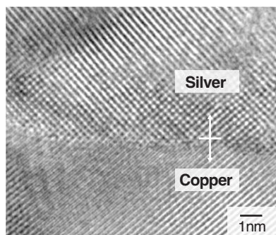
銀ナノ粒子を用いた新規低温焼結接合
