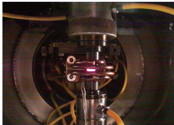
■超高温での力学特性評価
