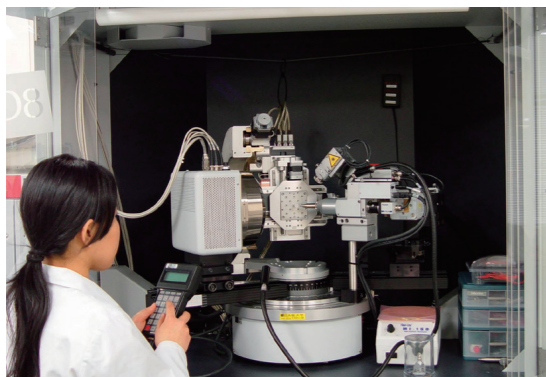
■微小領域X線回折装置。骨を含む結晶性材料の相同定や集合組織の解析を可能とします。
