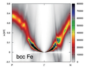
■図3:BCC鉄中のスピン波動起分散関係
