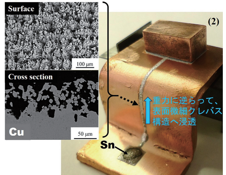
■(1) 銅などの金属表面へレーザーを照射すると、金属が3次元的に入り組んだ構造を持つ“表面微細クレバス構造”を局部的に作製できる。 ■(2) 表面微細クレバス構造に液体金属を接触させると“特異拡張濡れ”が発現する。液体金属は表面微細クレバス構造へ重力に逆らって浸透し、上部に置いた銅板と下銅板を接合させる。
