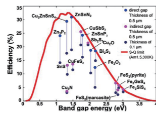
■図2:太陽電池材料のShockley-Queisser理論による効率予測
