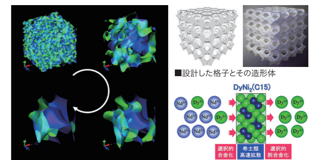
■規則ドメイン成長過程のフェーズフィールドシミュレーション ■合金の高度な選択透過性
