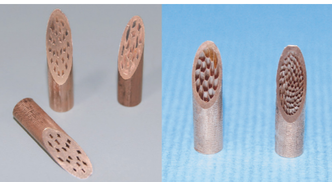
■固相接合を用いた新加工プロセスによる高強度ポーラス鋼
