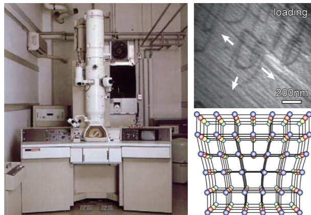
■透過型電子顕微鏡を用いた転位運動のその場観察
