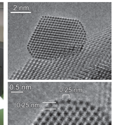
■触媒として気体分子と相互作用している金属ナノ粒子
